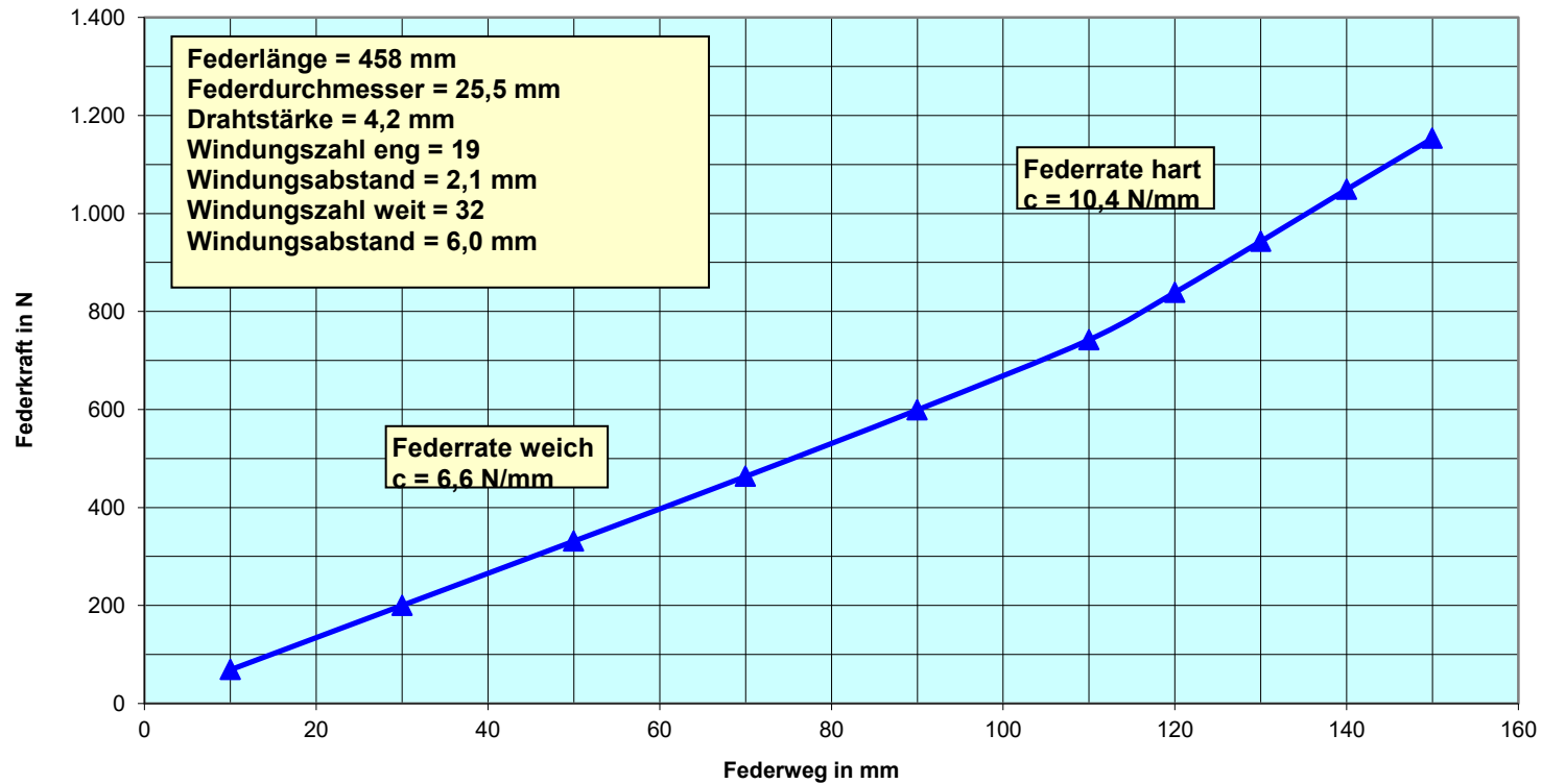
Kennlinie progressive Gabelfeder
